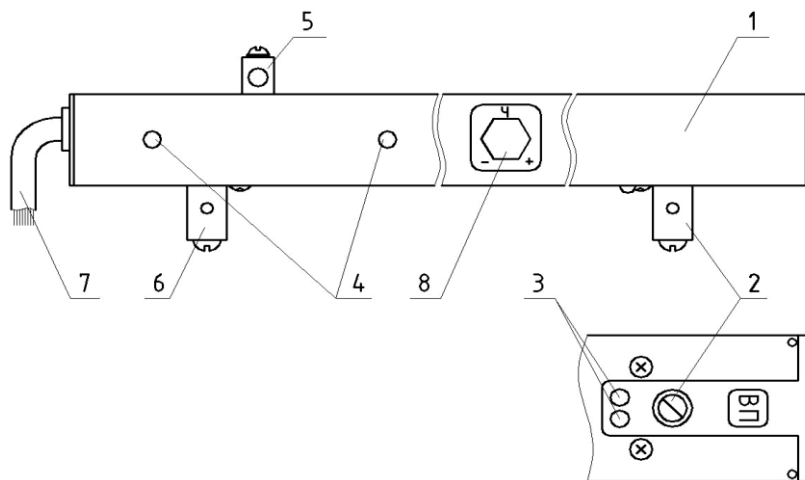
Рисунок 1.3 Конструкция ПРМ.
